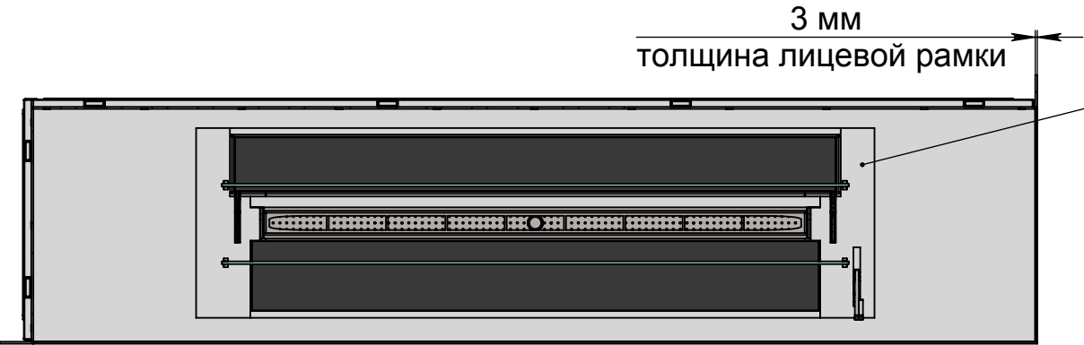
A-A (1 : 10)
